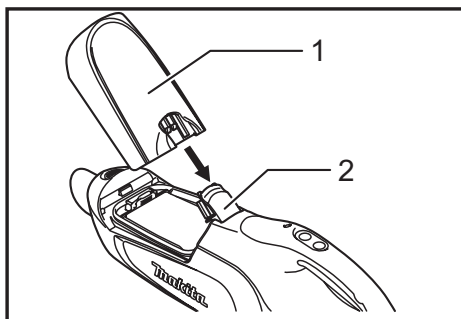
► 1. Couverture 2. Joint du couvercle avant
