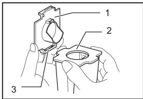
► 1. Tope para polvo 2. Filtro de papel 3. Ranura
