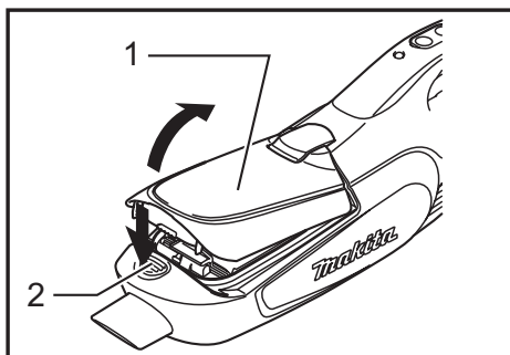
► 1. Couverture 2. Bouton
