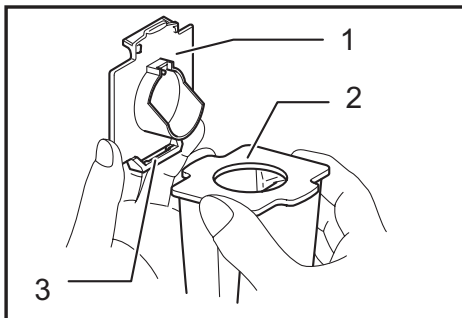
► 1. Pare-poussière 2. Filtre en papier 3. Rainure
